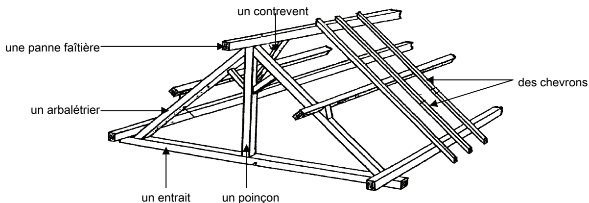
Schéma n°1 : assemblage d'une charpente classique
