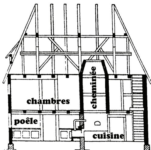
Schéma n°2 : charpente de la ferme de Recouvrance
