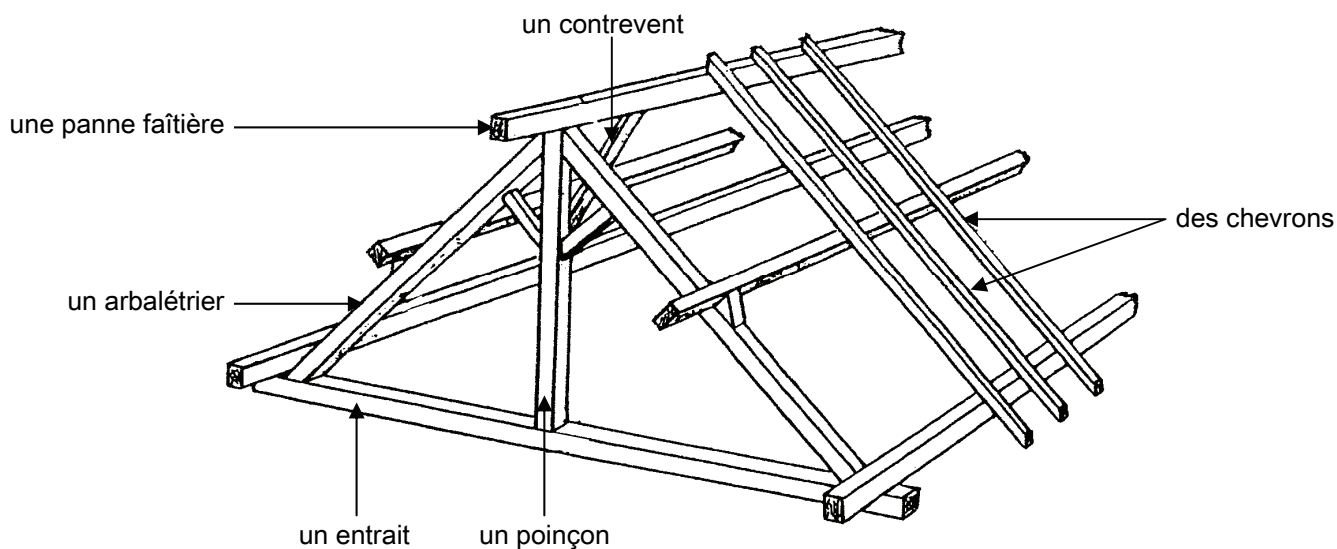
Schéma n°1 : assemblage d'une charpente classique
