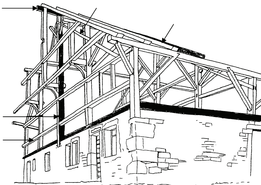
Schéma n°2 : charpente de la ferme des Arces-de-Morteau
